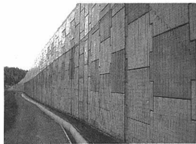
横浜市資源循環局(上)と国交省 山形河川国道事務所での施工例
